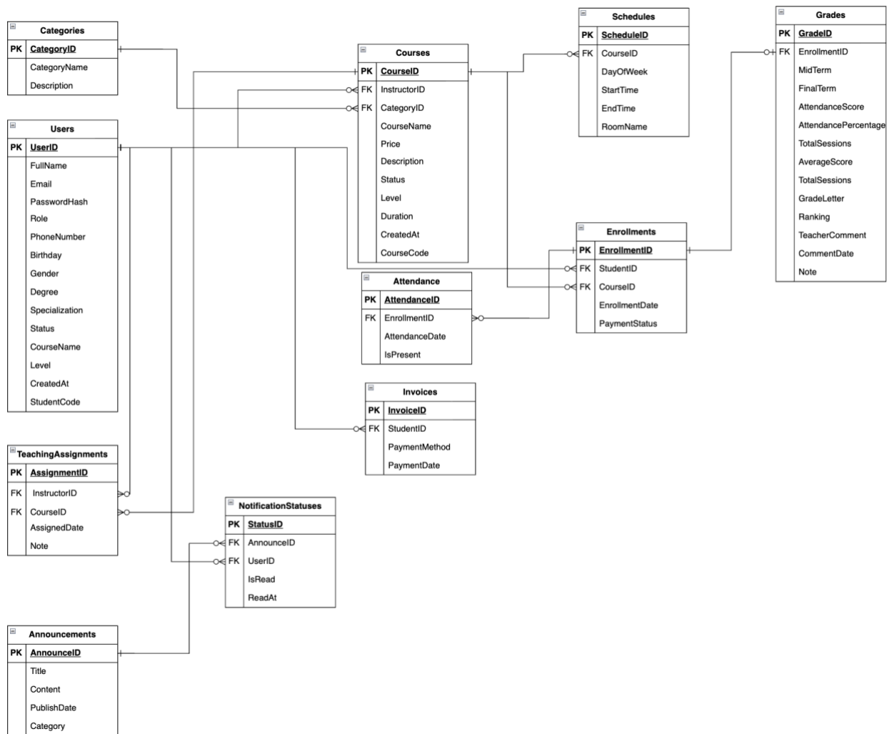
Hình 2. Sơ đồ Entity Relationship Diagram (Crow's Foot)
