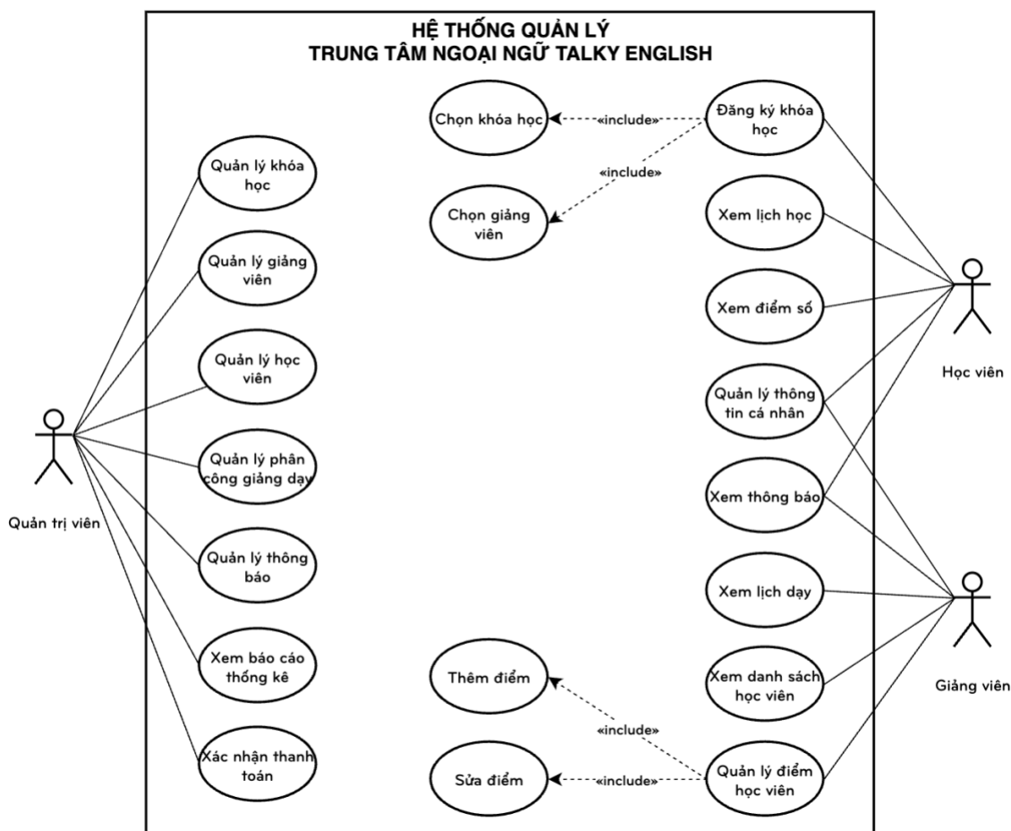
Hình 1. Sơ đồ Use Case tổng quan
